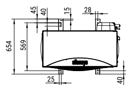
TOP VIEW VISTA EN PLANTA
