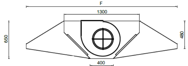
Modelo Central Vent 400°/2h
